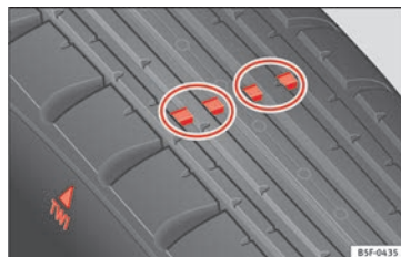
Obr. 189 Ukazatel opotřebení profilu pneumatiky
