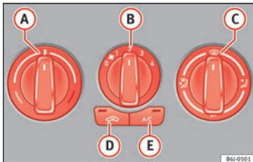
Obr. 49 Na středové konzole: Manuální ovládací prvky klimatizace
