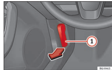
Obr. 6 Odjišťovací páčka v prostoru pro nohy řidiče.
