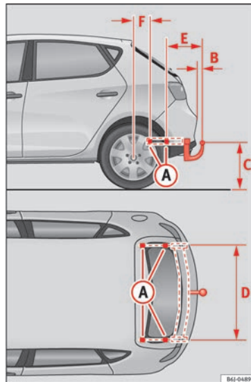
Obr. 184 IBIZA/IBIZA SC: Body k upevnění tažného zařízení
