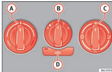
Obr. 50 Na středové konzole: Ovládací prvky systému vytápěného a čerstvého vzduchu
