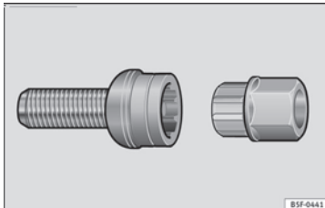
Obr. 64 Bezpečnostní šrouby kola s krytkou a adaptérem
