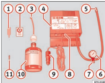
Obr. 60 Standardní zobrazení: Součásti opravárenské sady.
