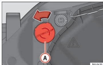
Obr. 103 Ukazatele směru jízdy (směrová světla)
