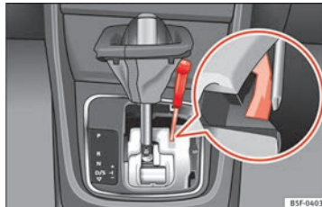
Obr. 55 Volicí páka: Nouzové odblokování z parkovací polohy
