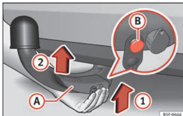
Obr. 222 Umístění odnímatelné kulové hlavy/odjišťovacích čepů v rozvinutém stavu
