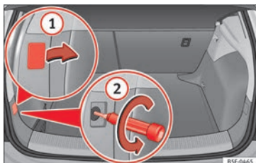
Obr. 115 Zavazadlový prostor: Poloha upevňovacího šroubu zadního světla
