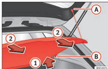
Obr. 158 Víko zavazadlového prostoru spolu s odkládacím příhrádkou je otevřeno.
