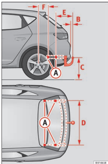
Obr. 231 Body k upevnění tažného zařízení
