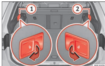
Obr. 151 V zavazadlovém prostoru: odjišťovací páčka ve vzdálenosti částí vlevo (1) a vpravo (2) od opěradla zadního sedadla.
