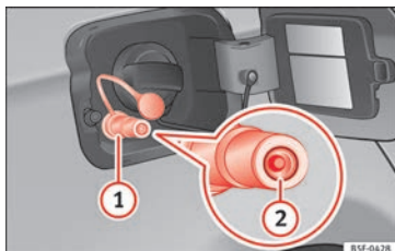
Obr. 232 Otevřené víko palivové nádrže: Plynové plnicí hrdlo ①, těsnicí kroužek plnicího hrdla ②.
