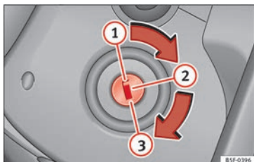
Obr. 184 Polohy klíče zapalování
