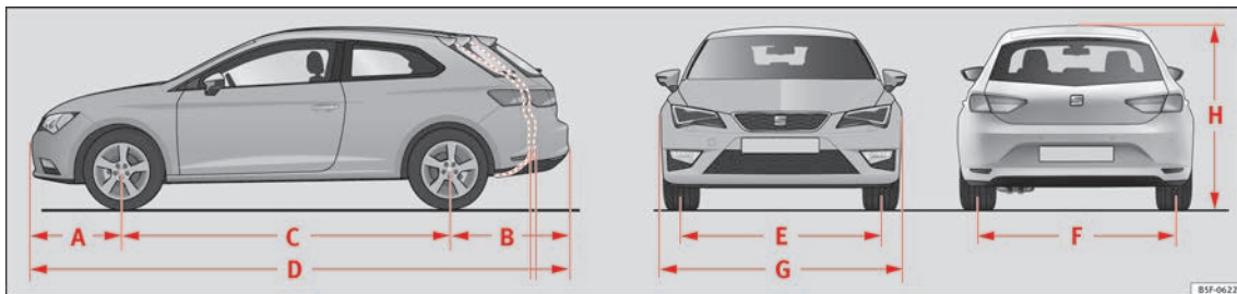
Obr. 243 Rozměry
