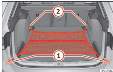
Obr. 175 V zavazadlovém prostoru: rovně zavěšená síť v zavazadlovém prostoru (model LEON ST).
