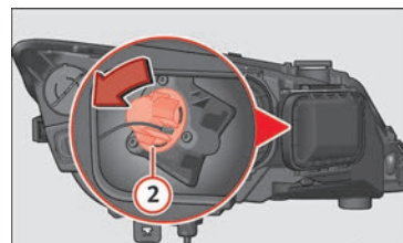
Obr. 107 Žárovka směrového světla
