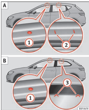
Obr. 181 Leon/Leon SC: Upevňovací body podélných tyčí střešních nosičů.
