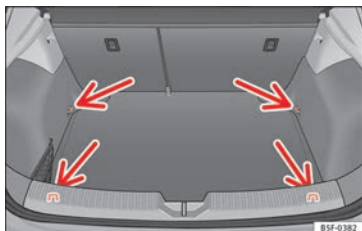
Obr. 171 V zavazadlovém prostoru: Vázací oka (model LEON/LEON SC mimo verzí s osazením náhradní pneu a GNC).
