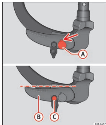
Obr. 221 Klidová poloha: poloha páky a odjišťovacích čepů
