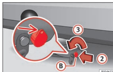
Obr. 227 Odblokování zámku
