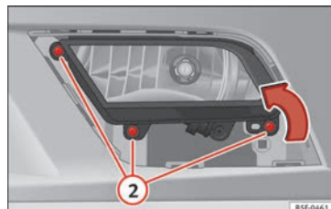
Obr. 111 Mlhové světlometry
