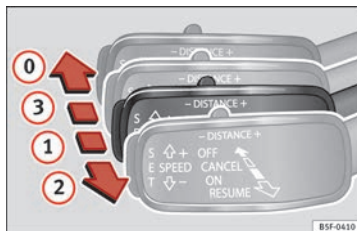
Obr. 195 Na levé straně sloupku řízení: třetí páčka pro ovládání automatické regulace odstupu.
