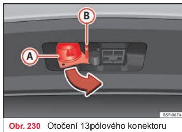
Obr. 230 Otočení 13pólového konektoru
