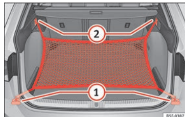
Obr. 176 V zavazadlovém prostoru: oka ① a háčky ② k zavěšení sítě v zavazadlovém prostoru (model LEON ST).
