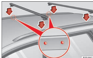
Obr. 182 Leon ST: Upevňovací body podélných tyčí střešních nosičů.
