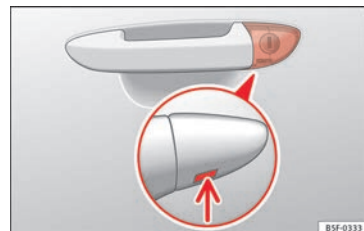
Obr. 3 Klička řidičových dveří: zapuštěná vložka zámku.
