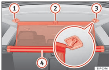
Obr. 165 V zavazadlovém prostoru: Zahákněte oddělovací síť.
