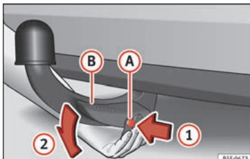
Obr. 228 Uvolnění odnímatelné kulové hlavy
