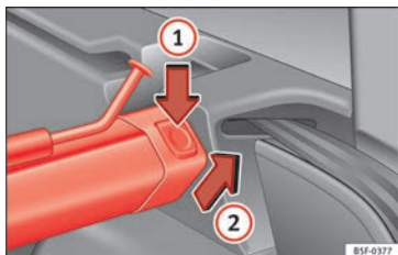
Obr. 166 V zavazadlovém prostoru: Demontujte oddělovací síť.
