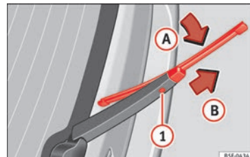
Obr. 82 Výměna lišty stěrače zadního skla.
