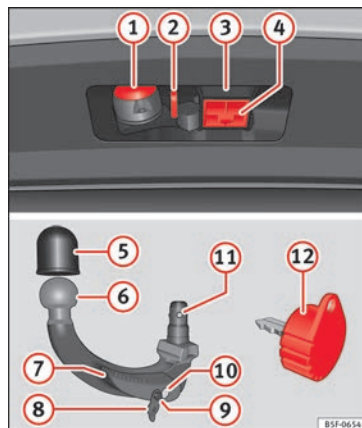
Obr. 218 Upevnění tažného zařízení/odnímatelná kulová hlava/klíč
