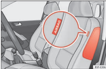
Obr. 26 Boční airbag v sedadle řidiče
