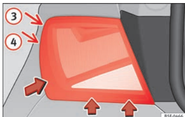
Obr. 116 Demontáž zadního světla v postranici
