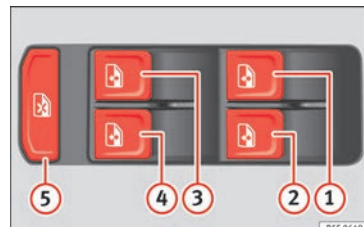
Obr. 136 Detail řidičových dveří: Ovládací tlačítka oken (vozidlo s 5 dveřmi a elektrickými spouštěči oken vpředu a vzadu).
