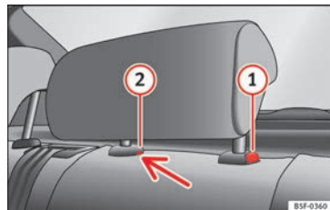
Obř. 145 Zadní opěrka hlavy uprostřed: Místo odblokování.
