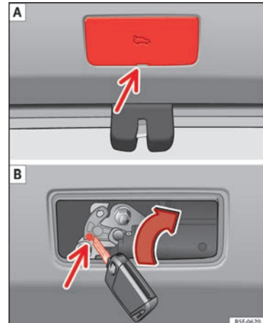
Obr. 7 Výřez zavazadlového prostoru: Přístup k nouzovému odemykání
