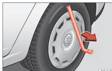
Obr. 69 Sejměte kryt kola z kola.
