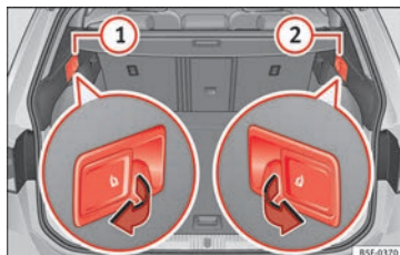
Obr. 152 V zavazadlovém prostoru: odjišťovací páčka ve vzdálenosti částí vlevo (1) a vpravo (2) od opěradla zadního sedadla.
