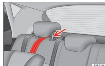
Obr. 33 Upevňovací pás: správné nastavení a správná montáž
