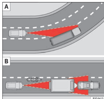
Obr. 205 (A) Vozidlo v zatáčce. (B) Řidič jedoucí na motorce před Vámi mimo rozpoznávací oblast radarového snímače.
