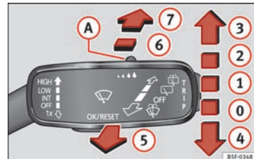
Obr. 39 Ovládání stěračů čelního a zadního skla
