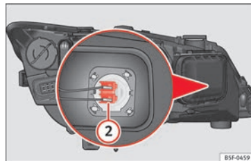
Obr. 108 Dálkové světlo.
