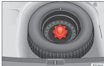
Obr. 248 Nouzové rezervní kolo: vyklápací dno ložného prostoru
