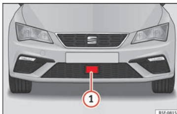
Obr. 208 V předním nárazníku: radarový snímač.
