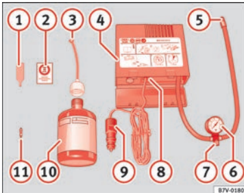
Obr. 67 Schématické zobrazení: Součásti opravárenské sady
