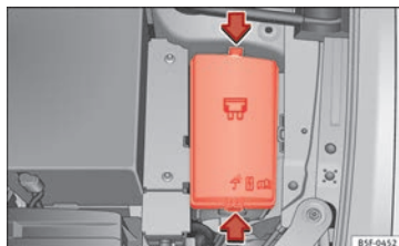
Obr. 101 V motorovém prostoru: kryt pojistkové skříňky.
