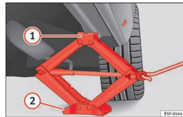
Obr. 74 Podélný nosník: nasazení zvedáku vozidla.
