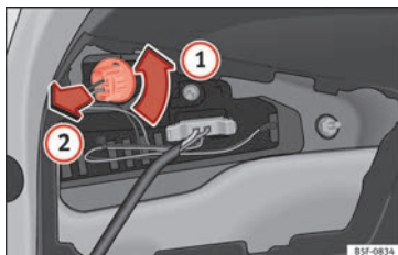
Obr. 116 demontujte držák žárovky.
