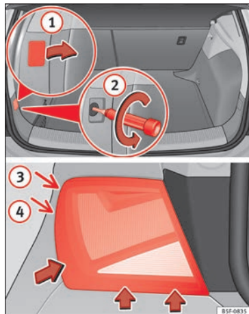
Obr. 111 Zavazadlový prostor: Poloha upevňovacího šroubu zadního světla demontáž zadního světla v postranici
