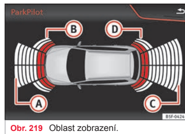
Obr. 219 Oblast zobrazení.
