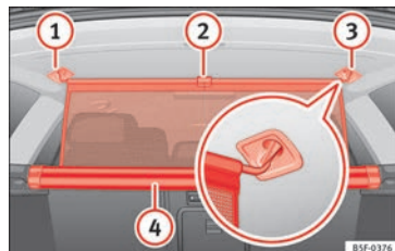
Obr. 167 V zavazadlovém prostoru: Zahákněte oddělovací síť.
