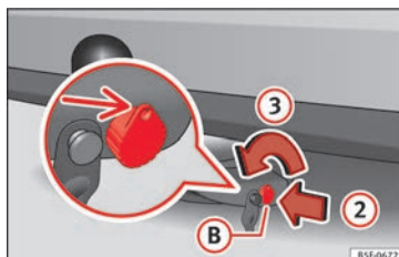
Obr. 234 Odblokování zámku
