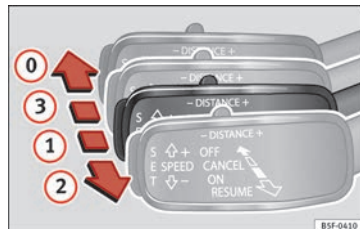
Obr. 200 Na levé straně sloupku řízení: třetí páčka pro ovládání automatické regulace odstupu.
