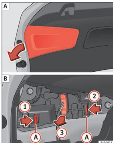
Obr. 113 Odstraňte kryt víka zavazadlového prostoru a demontujte nosič žárovky.
