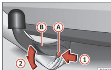
Obr. 235 Uvolnění odnímatelné kulové hlavy
