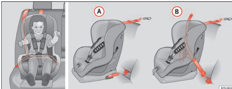
Obr. 30 Na zadních sedadlech: možná montáž dětských autosedaček.
