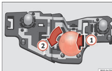
Obr. 114 Poloha žárovek na nosiči žárovek.
