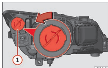
Obr. 104 Světlo denního svícení.
