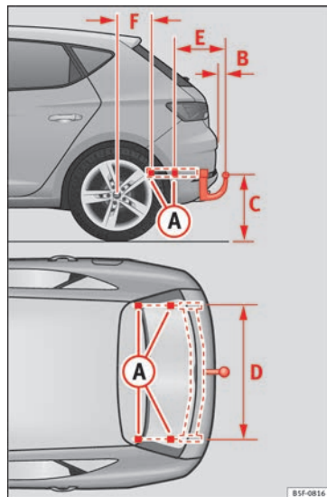
Obr. 238 Body k upevnění tažného zařízení
