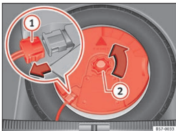
Obr. 249 V zavazadlovém prostoru: demontujte subwoofer.
