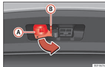
Obr. 237 Otočení 13pólového konektoru
