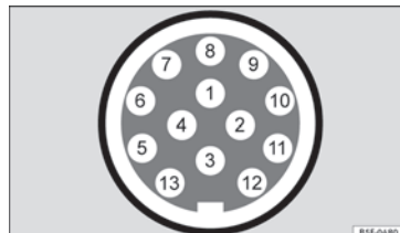
Obr. 236 Schématické zobrazení: Přirazení konektorových kolíků pro napájení přívěsu.
