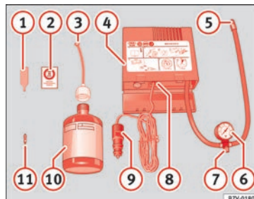
Obr. 96 Schématické zobrazení: Součásti opravářenské sady
