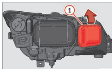
Obr. 107 Dálkové světlo.
