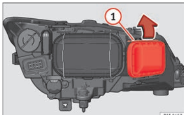
Obr. 105 Žárovka směrového světla
