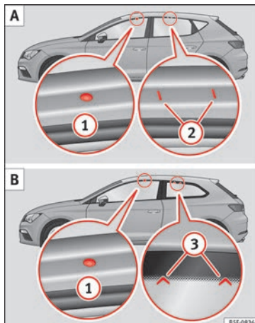
Obr. 183 Leon/Leon SC: Upevňovací body podélných tyčí střešních nosičů.
