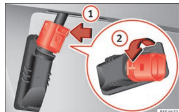
Obr. 118 Světlo registrační značky: Demontáž nosiče žárovky.
