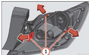
Obr. 112 Upevňovací spony zadní strany zadního světla.
