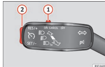
Obr. 47 Vlevo od sloupku řízení: Spínač a ovládací prvky tempomatu.
