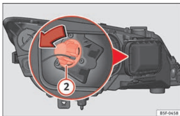
Obr. 106 Žárovka směrového světla
