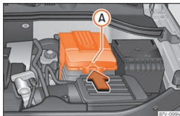
Obr. 298 V motorovém prostoru: sejmete kryt akumulátoru vozidla.
