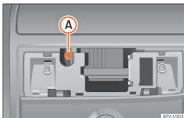
Obr. 18 Šroub s vnitřním šestihranem pro zavření panoramatické posuvné střešy
