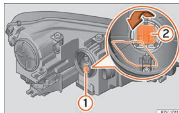
Obr. 110 držák žárovky ukazatele směru jízdy (1) a držák žárovky obrýsového světla (2)
