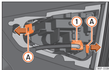
Obr. 62 demontujte držák žárovky.
