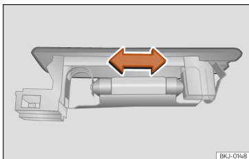
Obr. 66 Svítlna zavazadlového prostoru*
