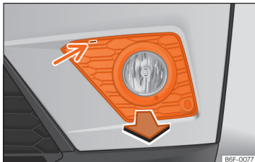
Obr. 57 Mlhový světlomet: vytažení mřížky
