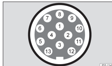
Obr. 262 Schématické zobrazení: Přístroje konektorových kolíků pro napájení přívěsu.
