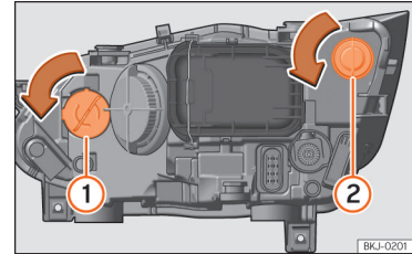
Obr. 56 V motorovém prostoru: žárovka směrového světla 1 a žárovka světla DRL (světla pro denní svícení) 2 .
