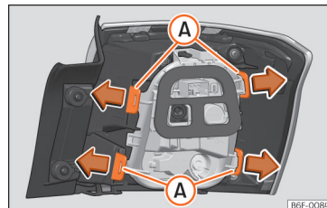
Obr. 60 Upevňovací spojky na zadní straně zadní svítilny.
