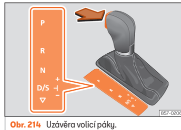
Obr. 214 Uzávěra volicí páky.
