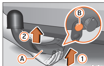
Obr. 266 Nasazení kulové hlavy - krok 1
