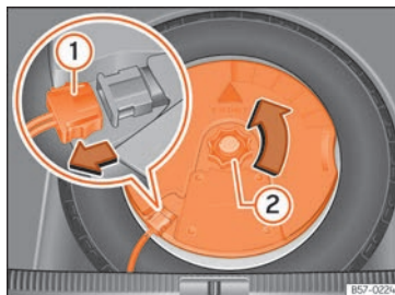
Obr. 285 V zavazadlovém prostoru: demontáž subwooferu.
