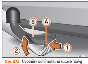
Obr. 272 Uvolnění odnímatelné kulové hlavy
