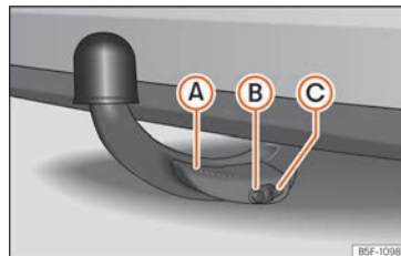
Obr. 269 Řádně upevněná odnímatelná kulová hlava
