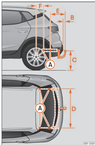
Obr. 275 Body k upevnění tažného zařízení
