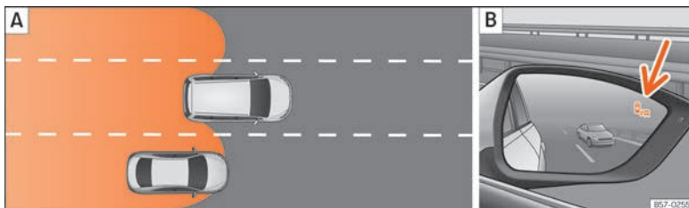
Obr. 244 Schématické zobrazení: [A] Předjíždění a následné zařazení do pravého jízdního pruhu. [B] Zobrazení asistenta mrtvého úhlu ve vnějším zrcátku vpravo.
