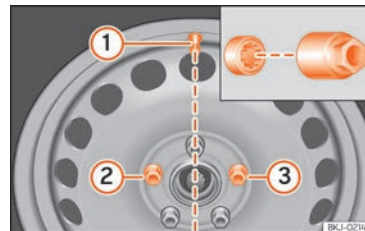
Obr. 73 Výměna kola: ventil pneumatiky ① a montážní polohy bezpečnostních šroubů kola ② nebo ③.
