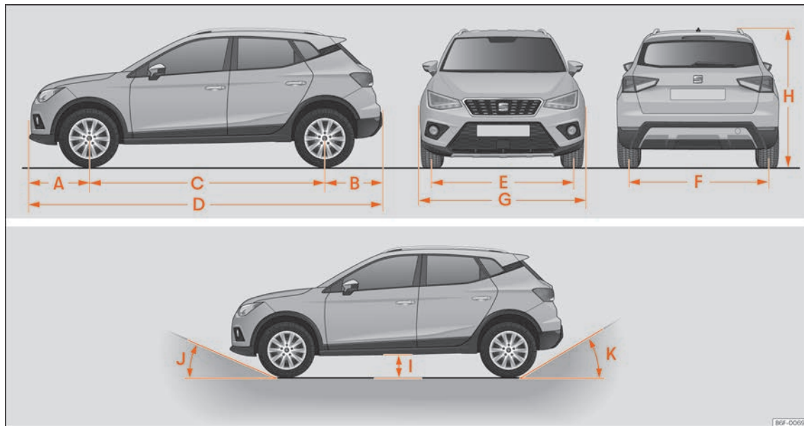
Obr. 287 Rozměry a úhly.
