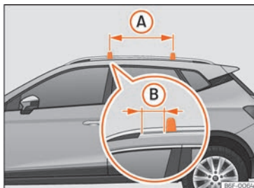
Obr. 166 Upevňovací body podélných nosníků pro střešní nosič zavazadel.
