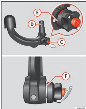
Obr. 197 Servisní poloha
