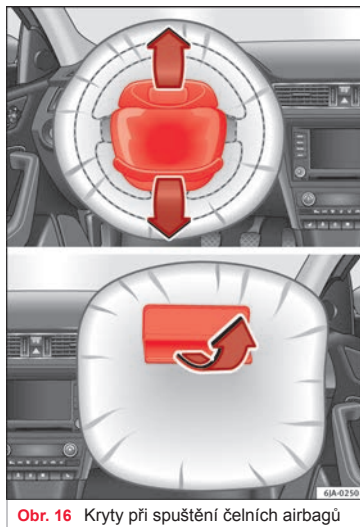
Obr. 16 Kryty při spuštění čelních airbagů
