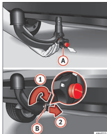
Obr. 198 Umístění tažné tyče/zavření zámku a vyjmutí klíče
