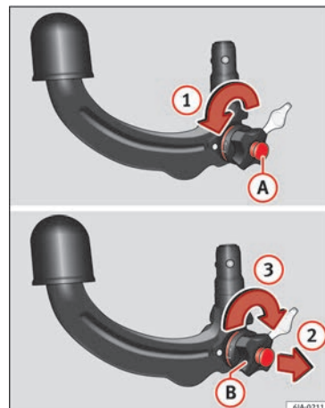
Obr. 196 Uvedení do servisní polohy
