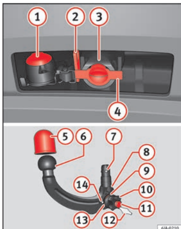
Obr. 195 Upevnění tažného zařízení/tažné tyče
