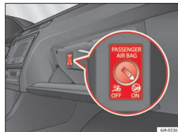
Obr. 17 Spínač čelního airbagu spolujezdce.
