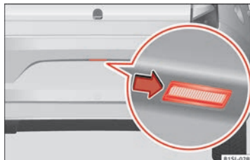
Obr. 90 Zadní nárazník: Demontujte světlo registrační značky.
