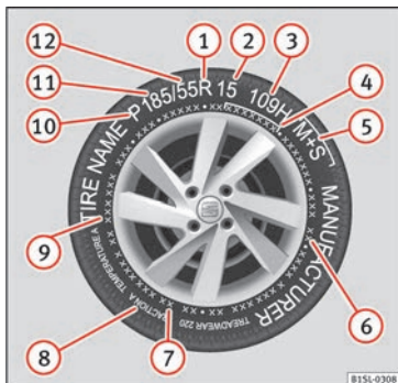
Obr. 177 Mezinárodní popis pneumatik
