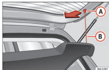
Obr. 133 V zavazadlovém prostoru: demontáž a montáž krytu zavazadlového prostoru.
