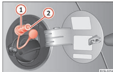
Obr. 166 Otevřené víko palivové nádrže: Plynové plnicí hrdlo ①, těsnicí kroužek plnicího hrdla ②.
