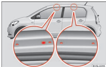
Obr. 138 Upevňovací body pro základní nosiče a nosiče zavazadel ve 4dvéřových vozidlech.
