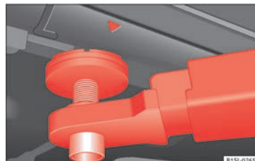
Obr. 159 Upevňovací body vzadu k zvedání vozidla zvedací plošinou nebo palubním zvedákem.
