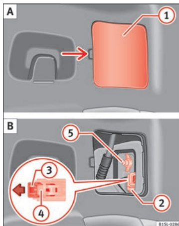
Obr. 88 Na straně v zavazadlovém prostoru: A: Sejmutí krytu, B: Demontáž zadního světla.
