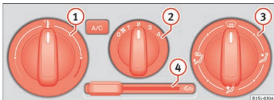
Obr. 140 Ve středové konzole: Ovládací prvky manuální klimatizace.
