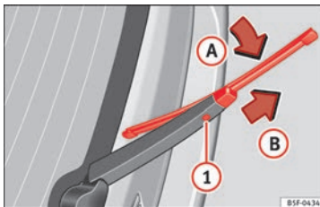
Obr. 63 Výměna lišty stěrače zadního skla.
