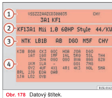
Obr. 178 Datový štítek.
