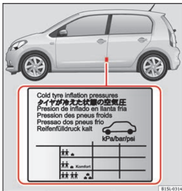
Obr. 173 Montážní poloha štítku tlaku vzduchu v pneumatikách.
