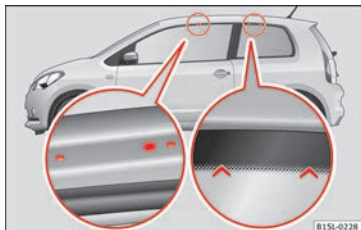
Obr. 137 Upevňovací body pro základní nosiče a nosiče zavazadel ve 2dvéřových vozidlech.
