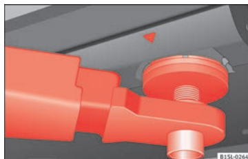
Obr. 158 Upevňovací body vpředu k zvedání vozidla zvedací plošinou nebo palubním zvedákem.
