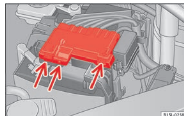
Obr. 171 V motorovém prostoru: sejměte kryt akumulátoru vozidla.
