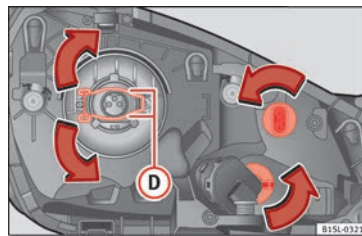
Obr. 85 Levý světlomet
