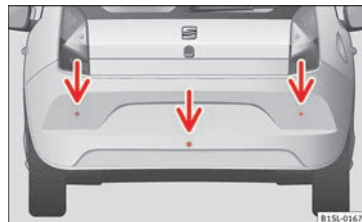
Obr. 148 Snímače kontroly odstupu při parkování v zadním nárazníku.
