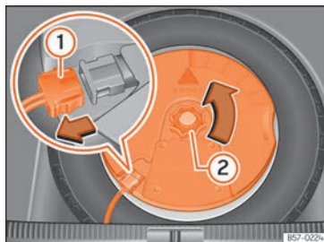
Obr. 275 V zavazadlovém prostoru: demontáž subwooferu.
