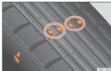
Obr. 272 Ukazatel opotřebení profilu pneumatiky
