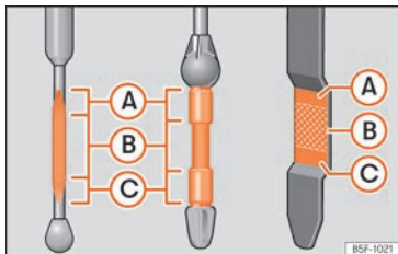
Obr. 270 Měrka oleje
