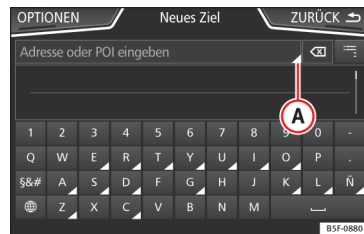
Obr. 43 Vyhledávací maska
